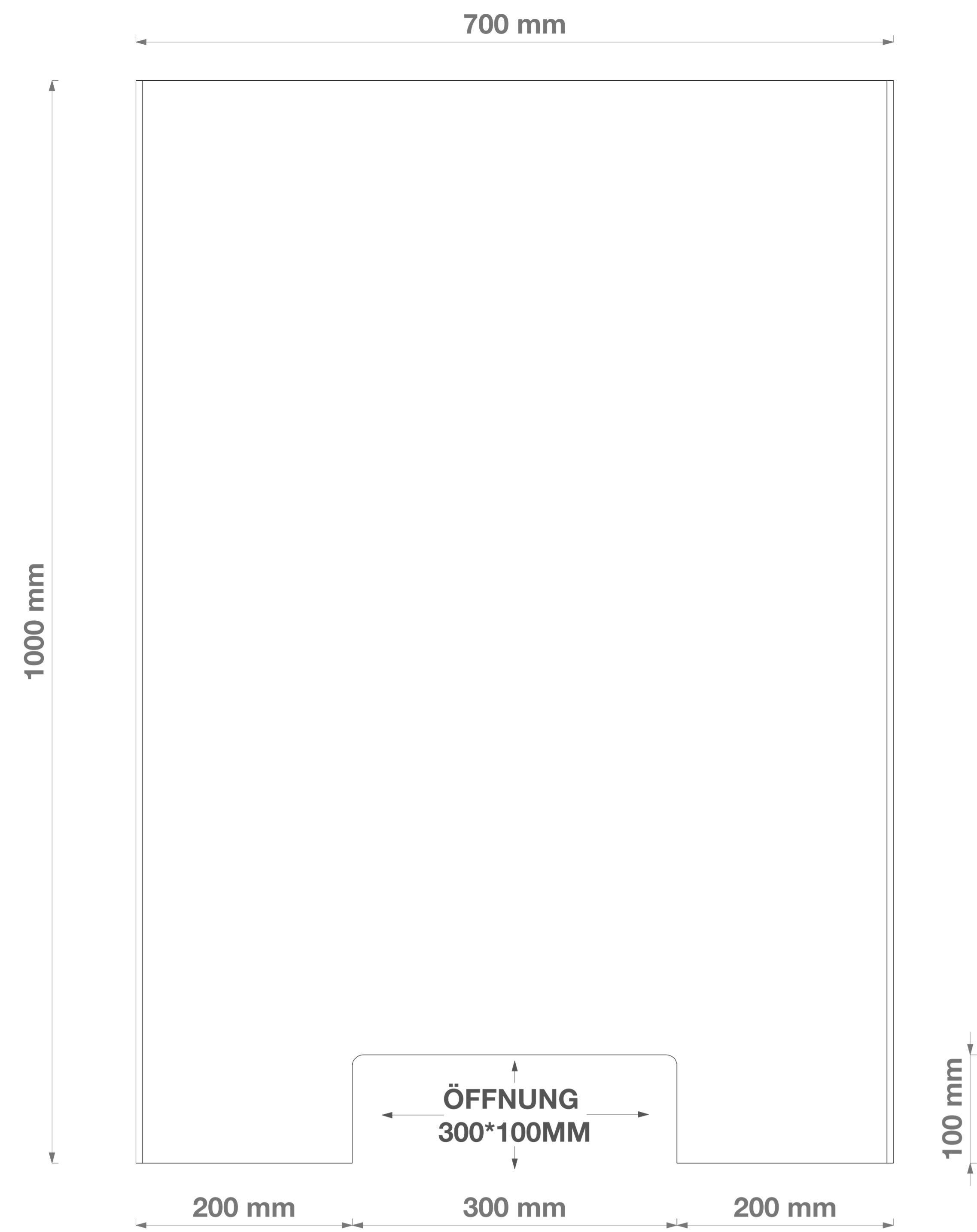
ANSICHT
